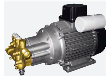
Elektrische Drei-Kolben-Axialpumpe mit Messingkopf Induktionsmotor mit Motorschutzschalter
